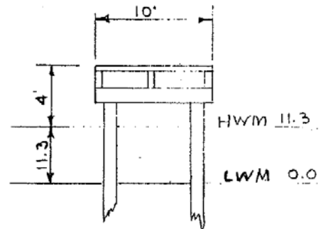
SECTION A-A SCALE: 1" = 10'
